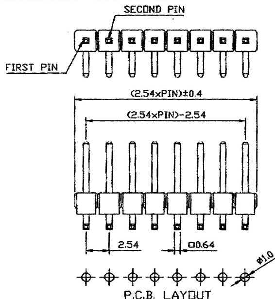
P.C.B. LAYOUT
